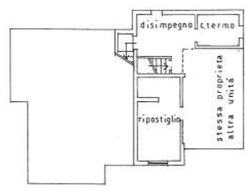
PIANTA PIANO TERRA H=2.03
