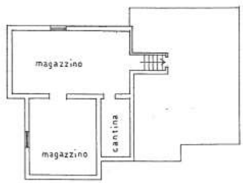
PIANTA PIANO SEMINTERRATO H=1.80
