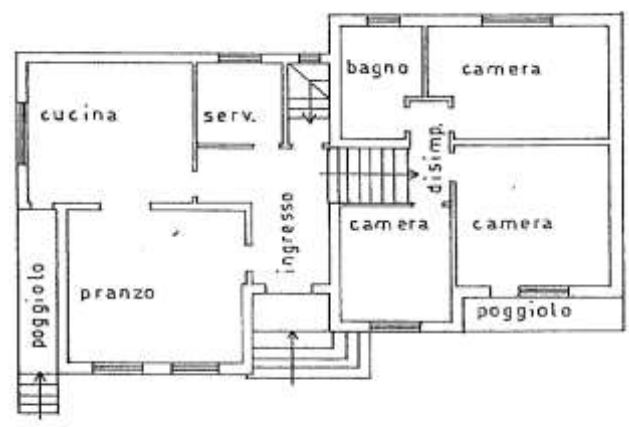
PIANTA PIANO PRIMO H=2.80
